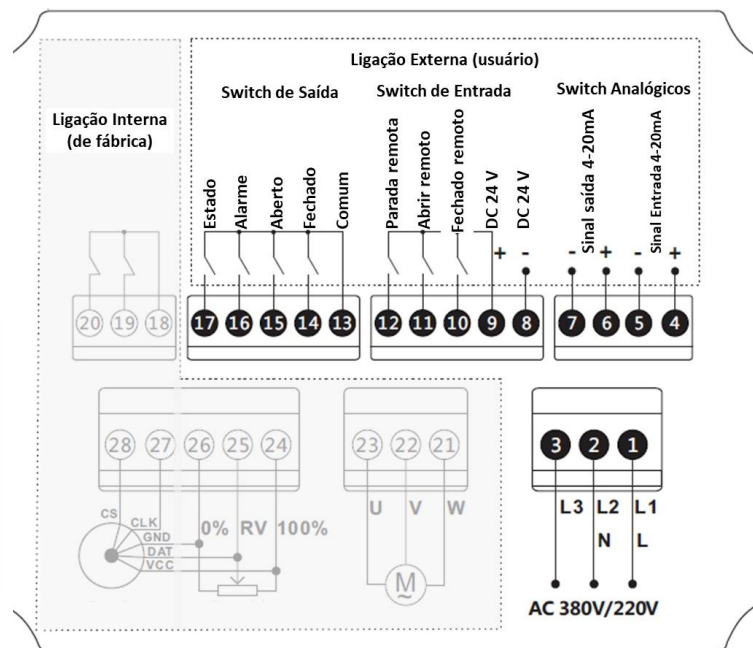
Diagrama versão AC
