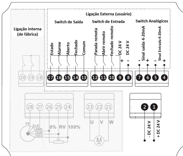
Diagrama versão DC
